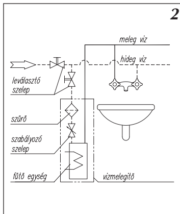
2. Ábra Vízrendszer bekötési vázlat
